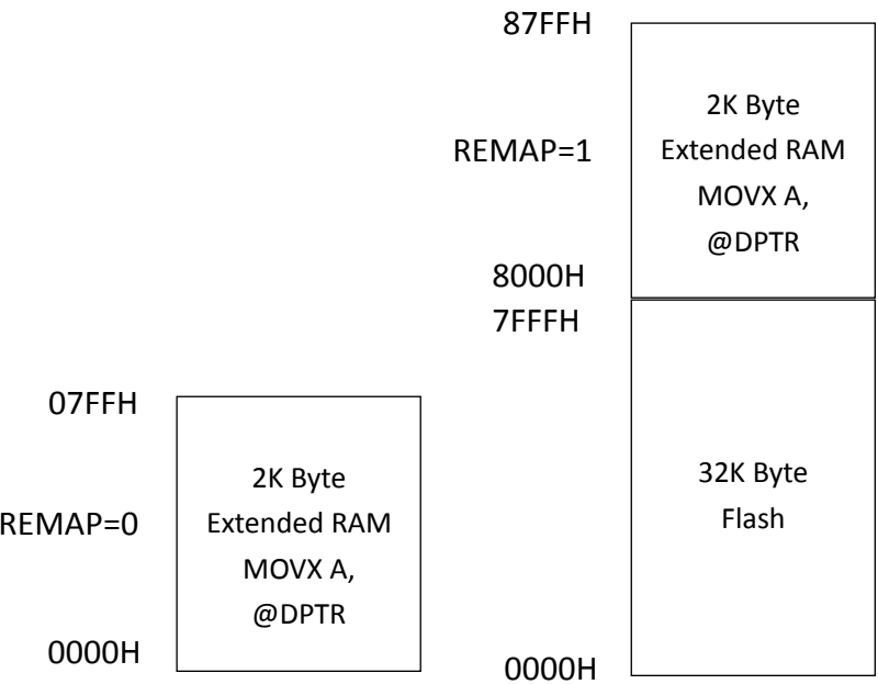
图 7-4-3 XRAM 地址映射图
