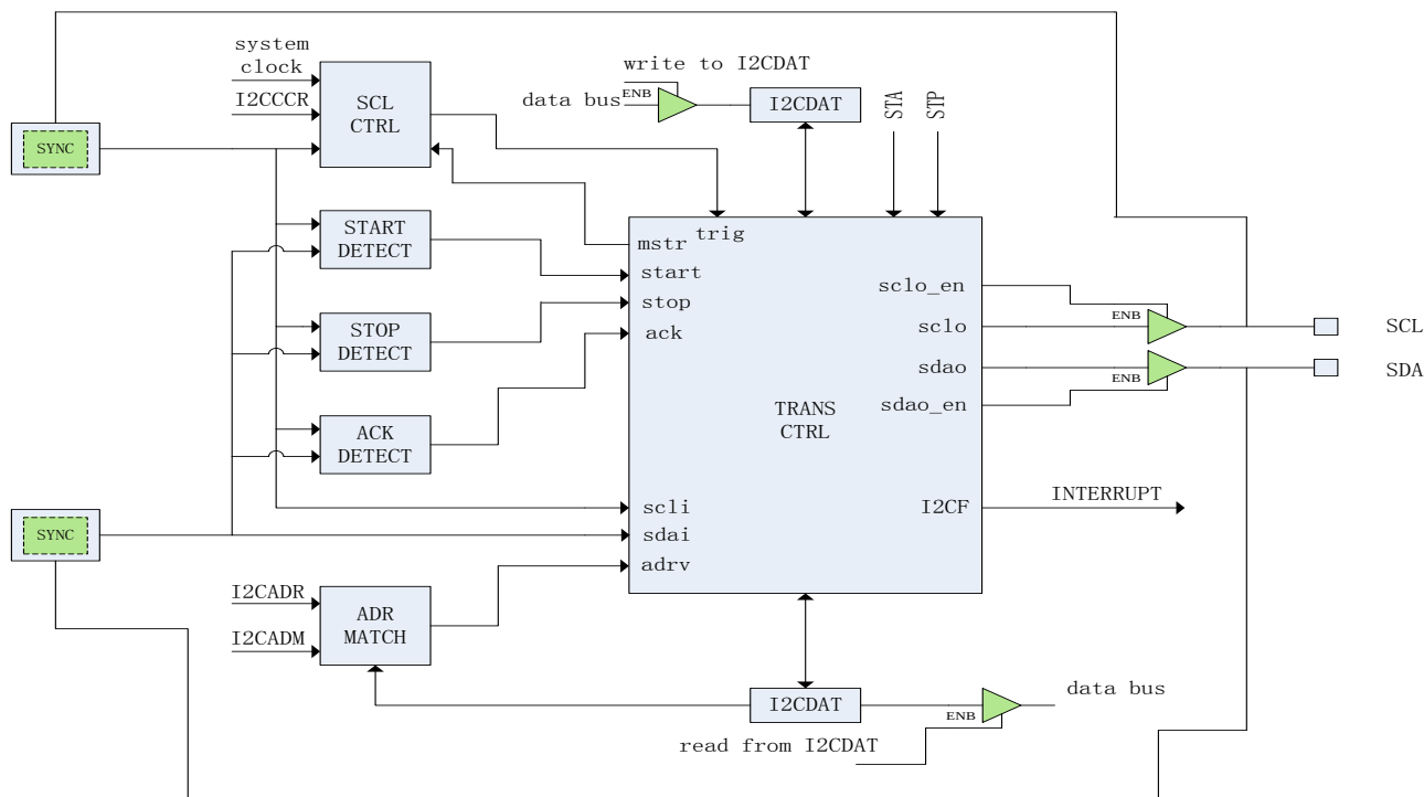
图 19-3-2 I²C 模块原理示意图
