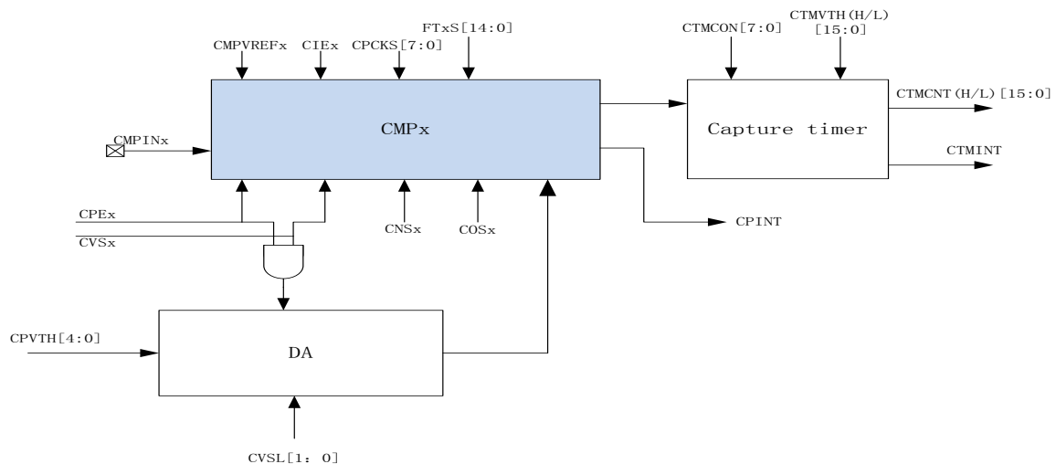
图 23-1-1 CMP 模块示意图
