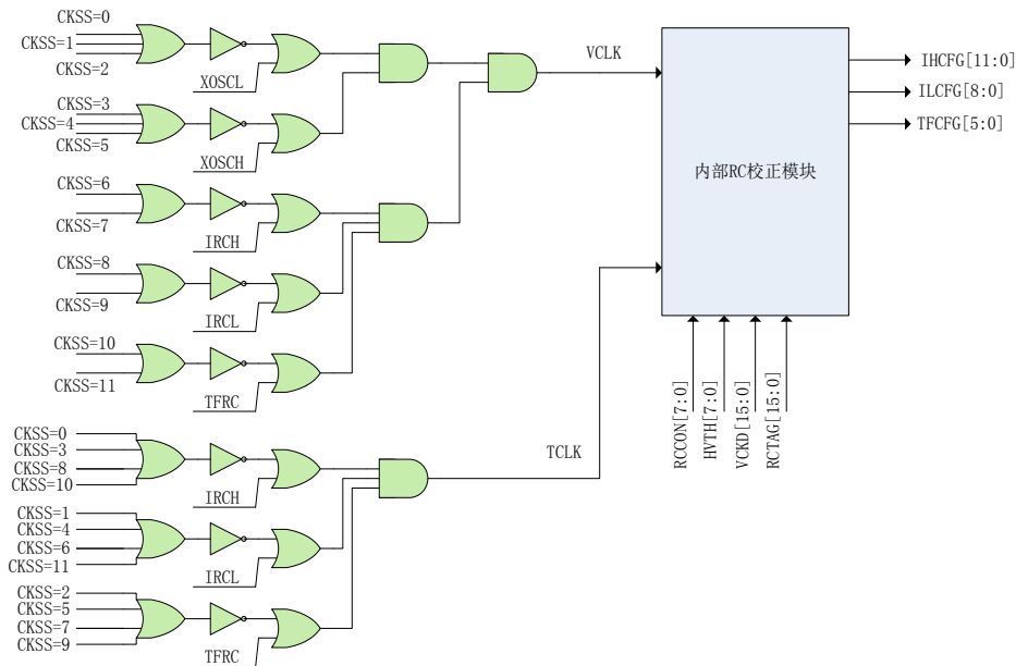
图 9-4-1 校正电路示意图
