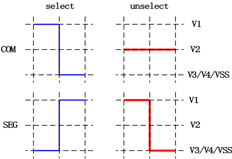
图 20-1-1-2 LCD 偏压比 1/2 信号
