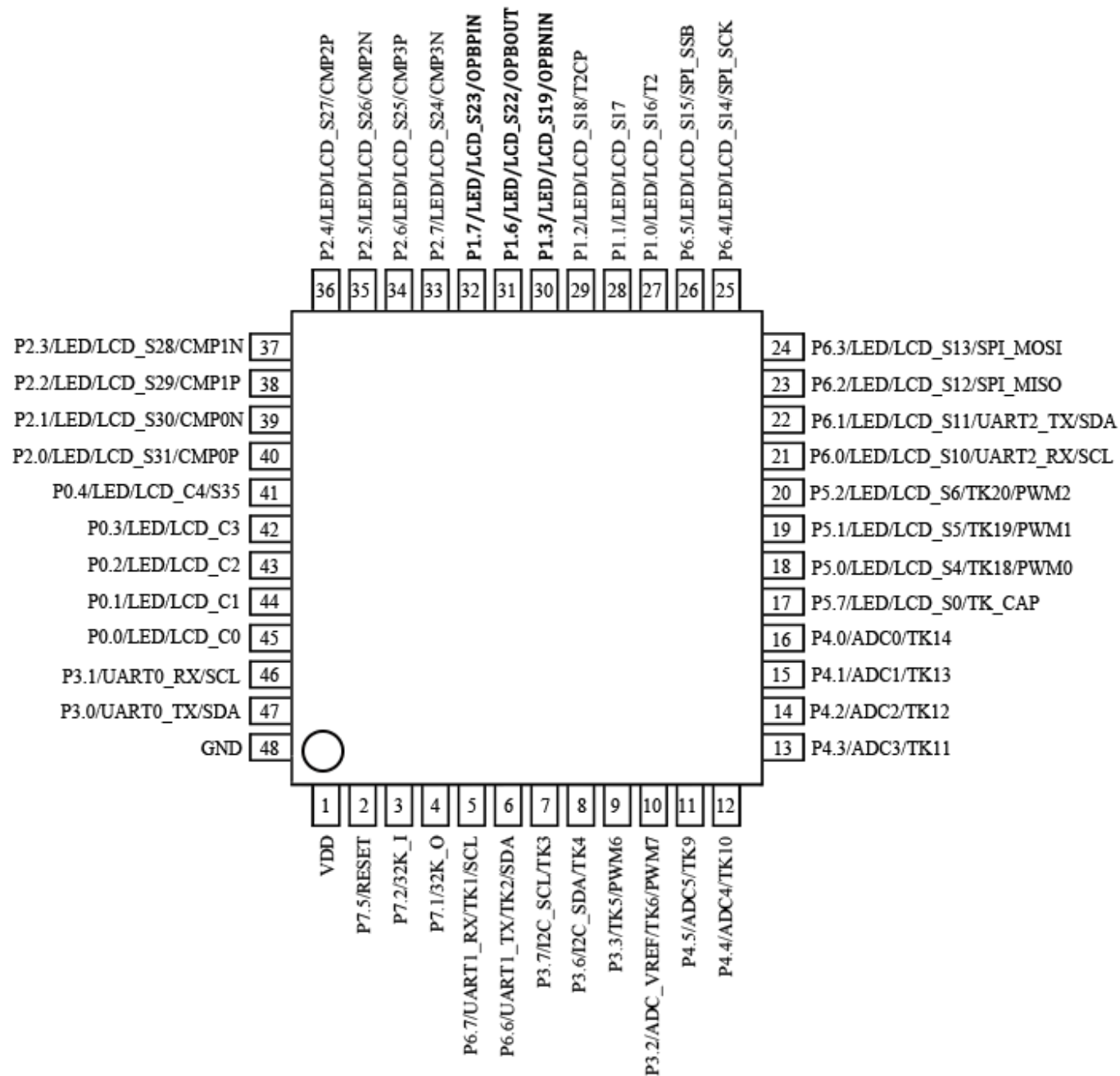
图 5-1-2 LQFP48 封装图
