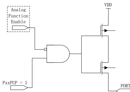
图 15-1-4 I/O 上拉模式结构示意图
