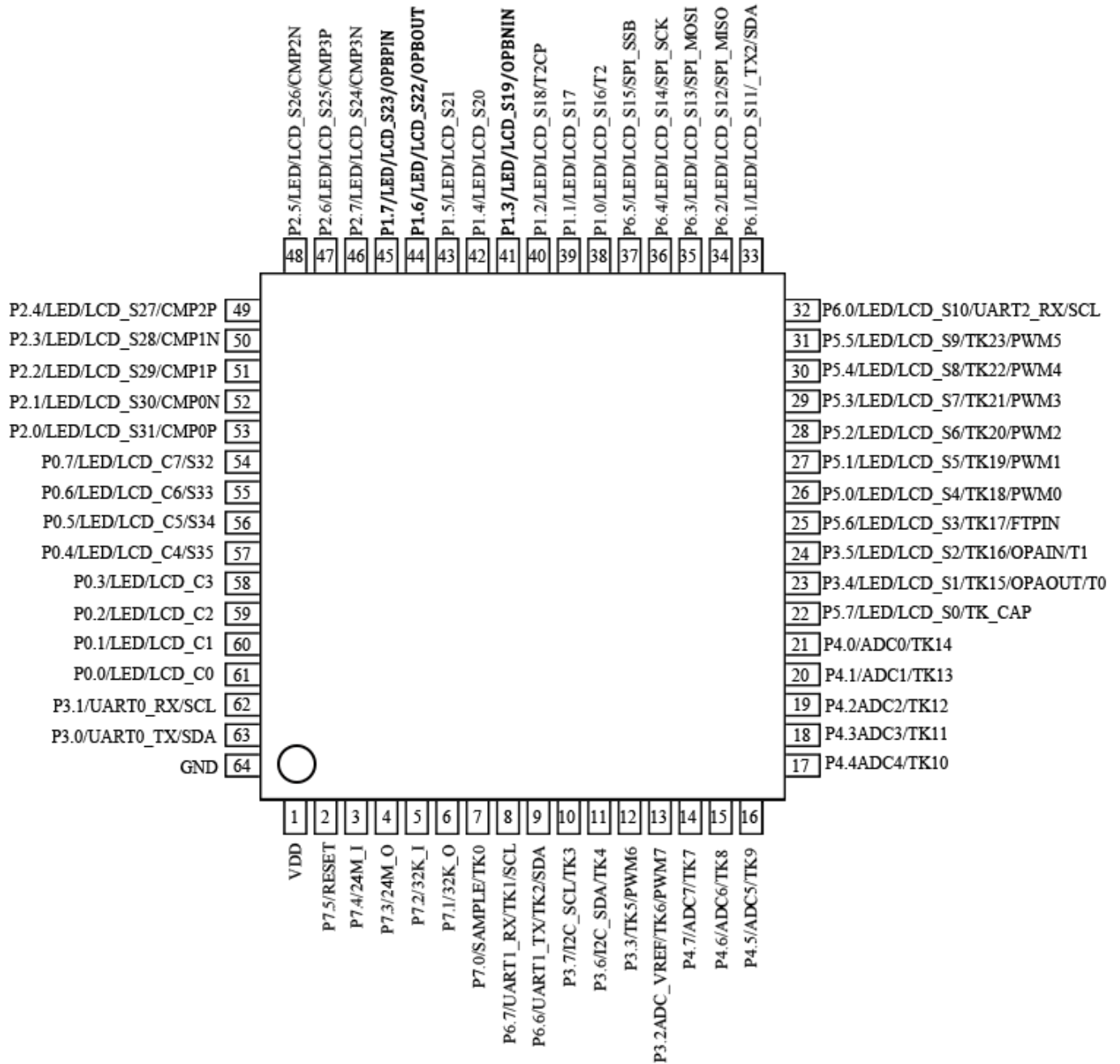
图 5-1-1 LQFP64 封装图
