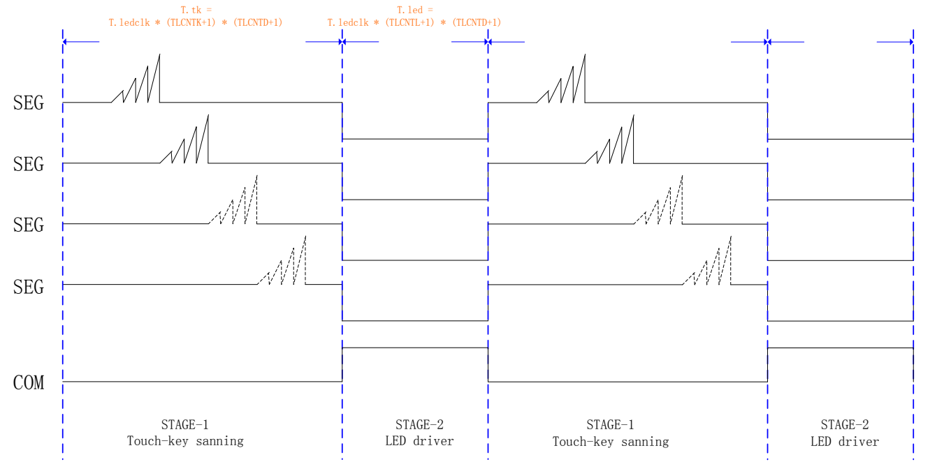
图 25-5-1 触摸共用 LED 驱动示意图
