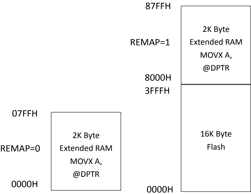
图 7-4-2 XRAM 地址映射图
