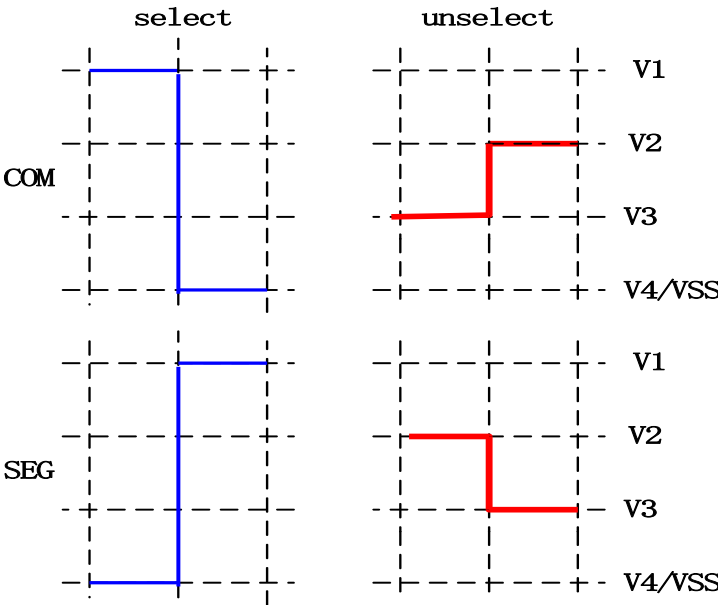
图 20-1-1-3 LCD 偏压比 1/3 信号
