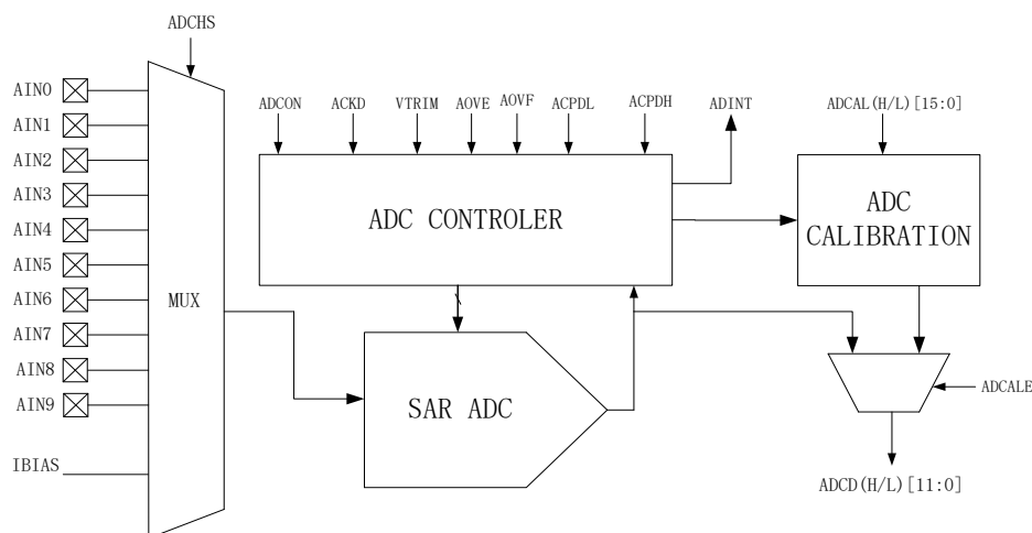
图 20-3-1 ADC 结构示意图
