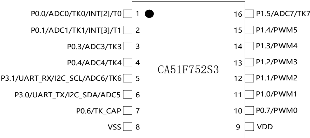
图 5-1-2 SOP16 封装图
