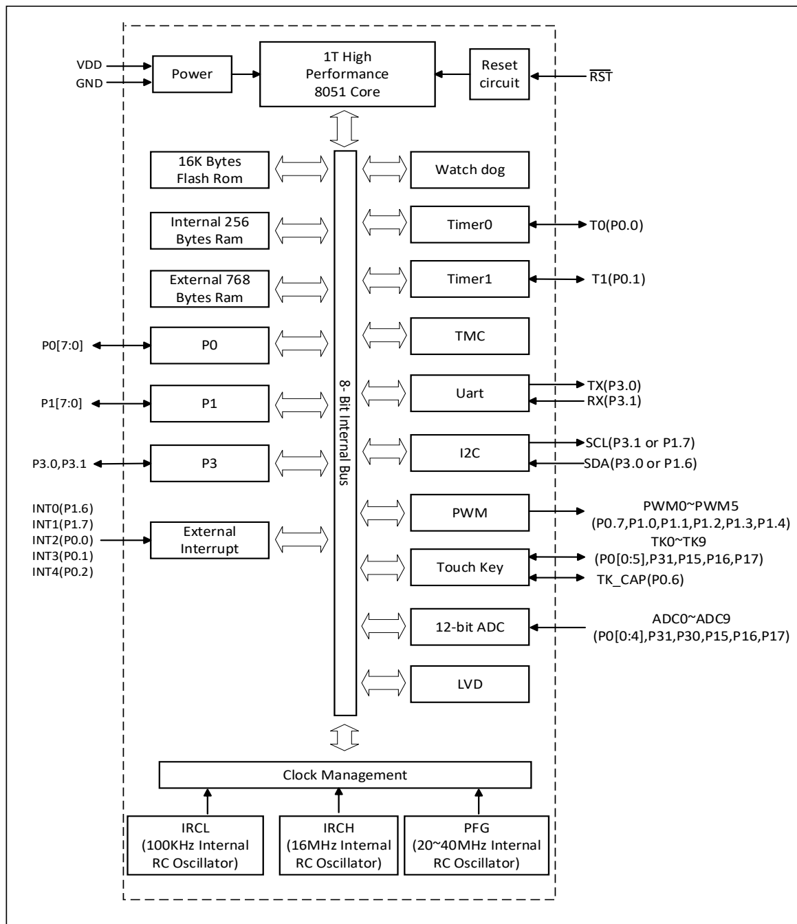
图 4-1-1 芯片框图
