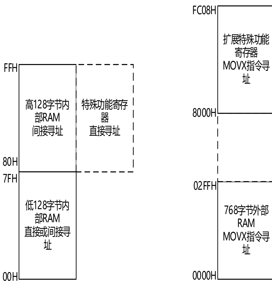
图 7-1-1 RAM 组织结构图
