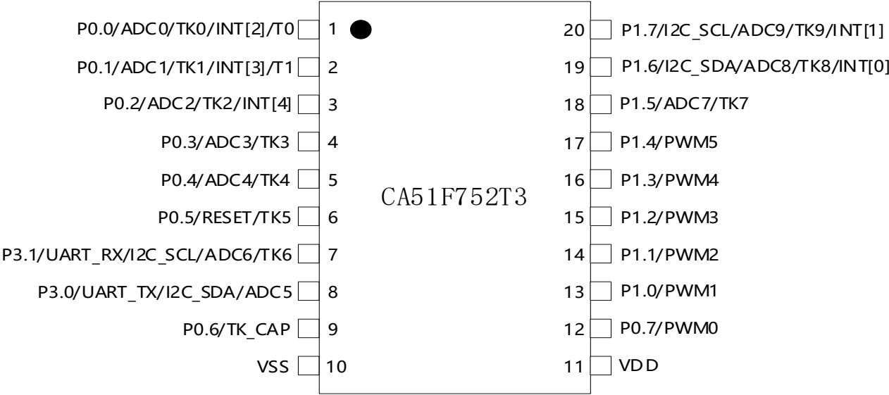
图 5-1-1 TSSOP20 封装图
